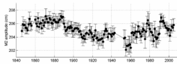
Fig. 1. Évolution de l'amplitude de l'onde de marée M2 à Brest (les barres d'erreur correspondent à \pm un écart-type).
