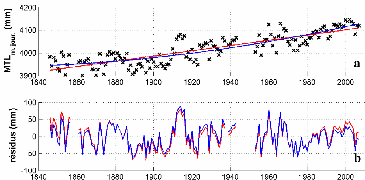
Fig. 8.3 – Les MTL_{m.jour.} à Brest entre 1846 et 2007. a : les MTL_{m.jour.} observées (régressions linéaire en rouge et quadratique en bleu) ; b : résidus ou écarts entre les moyennes observées et les courbes de régression (même convention de couleur).
