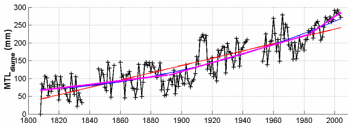
Fig. 8.17 – Moyennes annuelles des niveaux moyens diurnes de la marée ( MTL_{diurnes} ) à Brest depuis 1807. La droite rouge correspond à la tendance linéaire et la courbe bleue prend en compte une accélération. Les droites violettes correspondent aux tendances calculées pour : 1807-1892, 1892-1983, 1983-2004.
