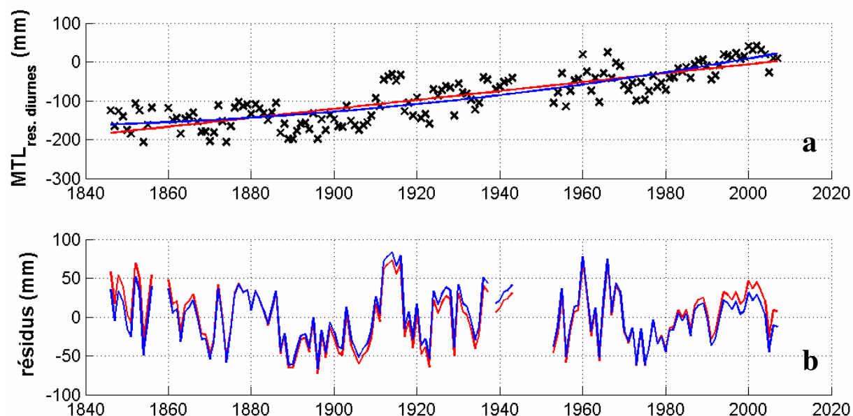
Fig. 8.7 – Les MHW rés. diurnes à Brest entre 1846 et 2007. a : les MHW rés. diurnes observées (régressions linéaire en rouge et quadratique en bleu) ; b : résidus ou écarts entre les moyennes observées et les courbes de régression (même convention de couleur).
