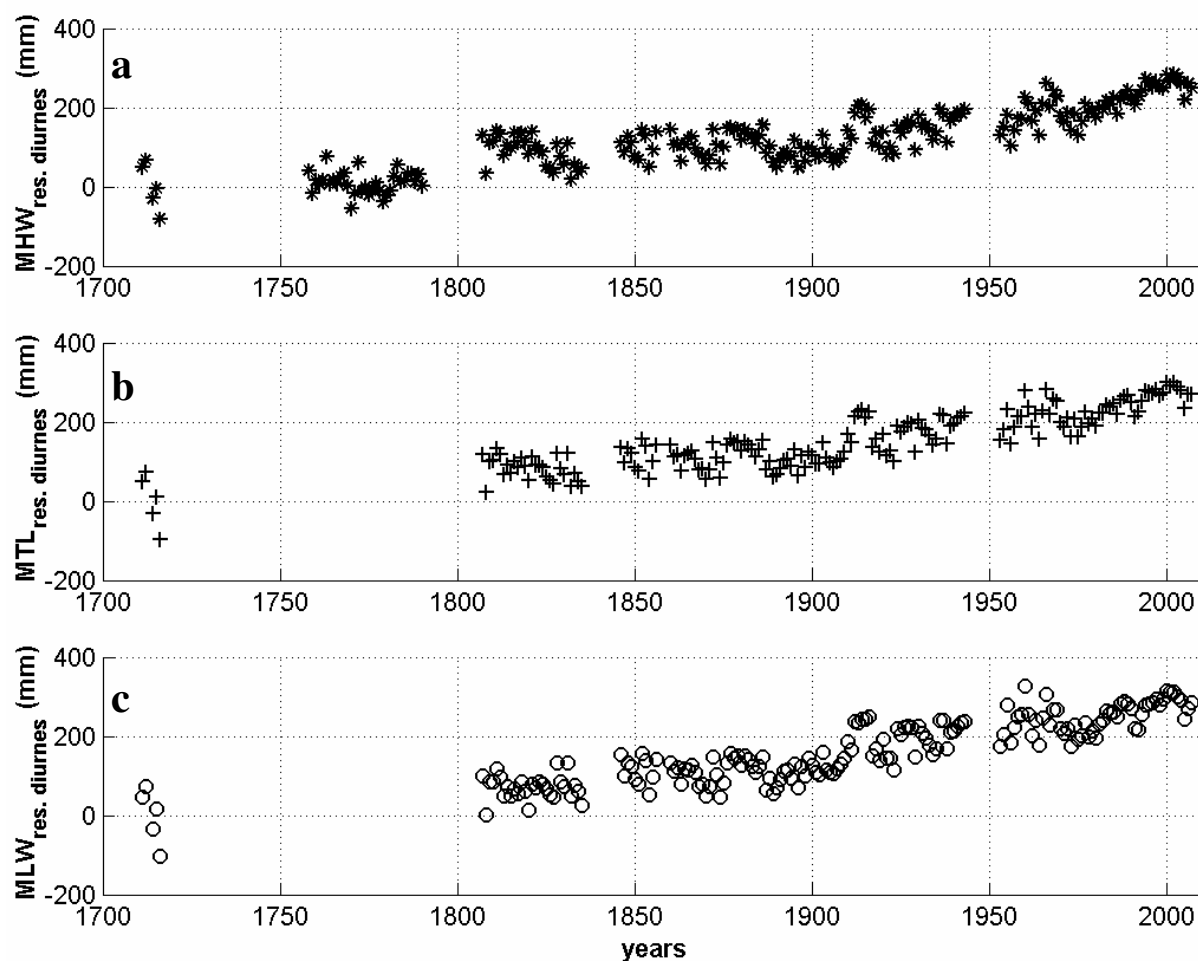
Fig. 8.12 – Moyennes annuelles des résidus à Brest depuis 1711 : a) pleines mer diurnes ( MHW_{res. diurnes} ) ; b) niveaux moyens diurnes de la marée ( MTL_{res. diurnes} ) ; c) basses mers diurnes ( MLW_{res. diurnes} ).
