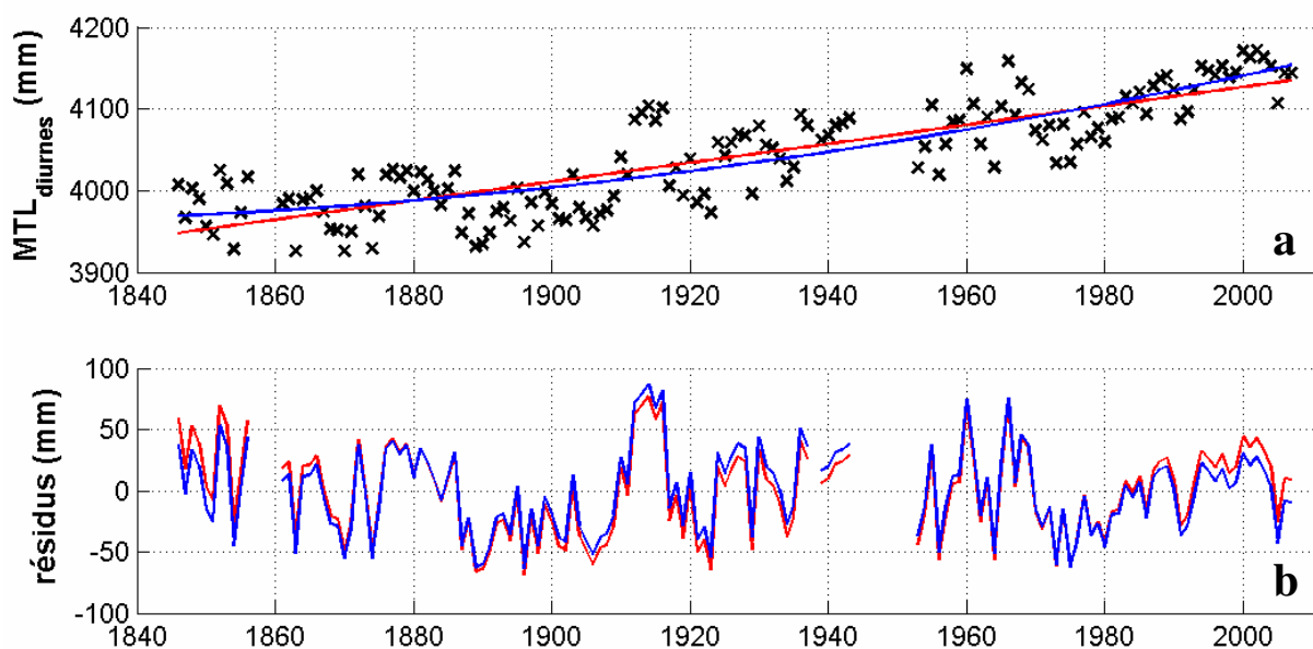
Fig. 8.4 – Les MTL_{diurnes.} à Brest entre 1846 et 2007. a : les MTL_{diurnes.} observées (régressions linéaire en rouge et quadratique en bleu) ; b : résidus ou écarts entre les moyennes observées et les courbes de régression (même convention de couleur).
