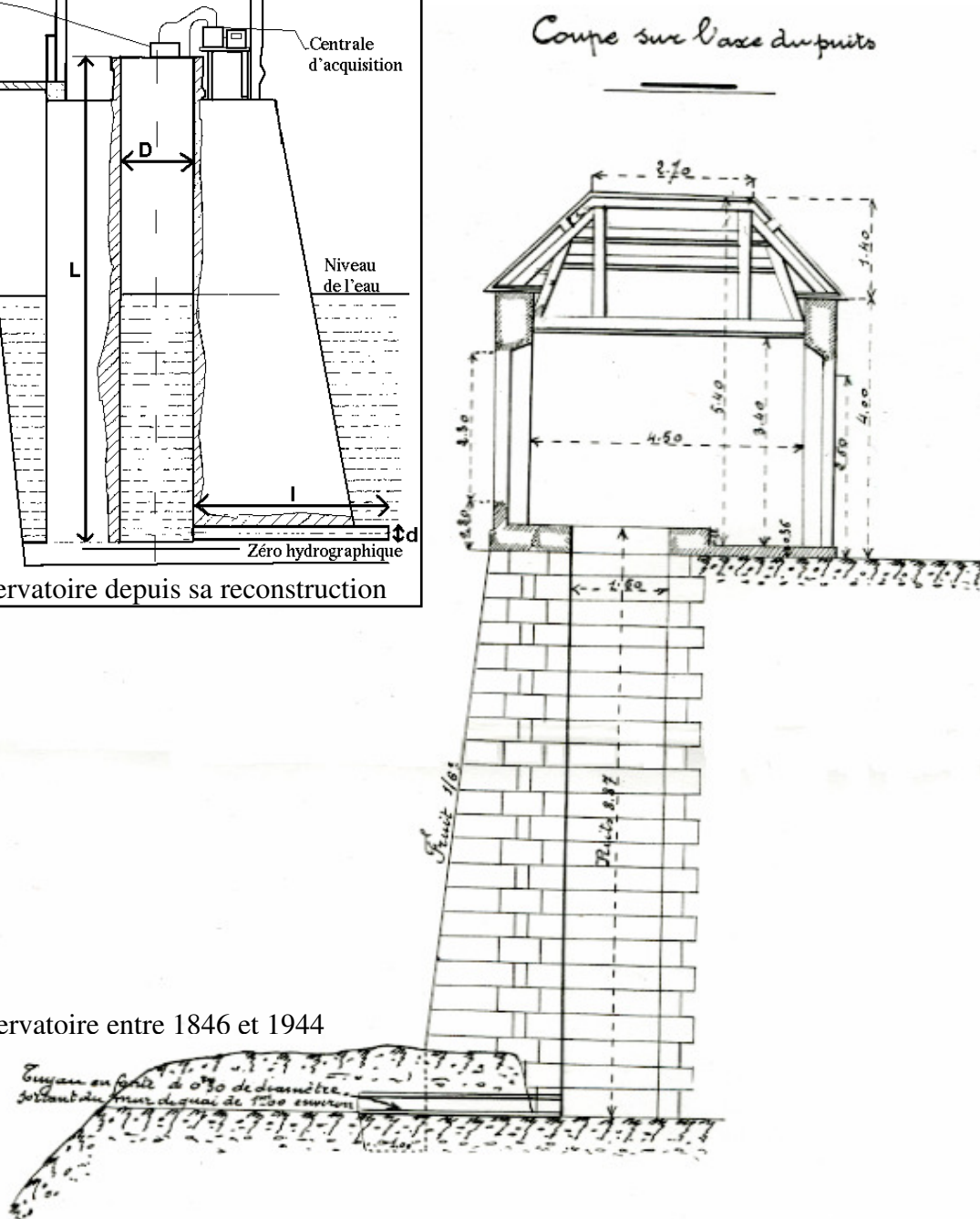
Fig. 6.12. – Schéma de l'Observatoire de Brest. Sources : a : Archives du SHOM, cote D818 ; b : modifié, d'après le SHOM. URL : http://www.shom.fr/fr_page/fr_act_oceano/img/brest.gif (consulté le 5 octobre 2008).
