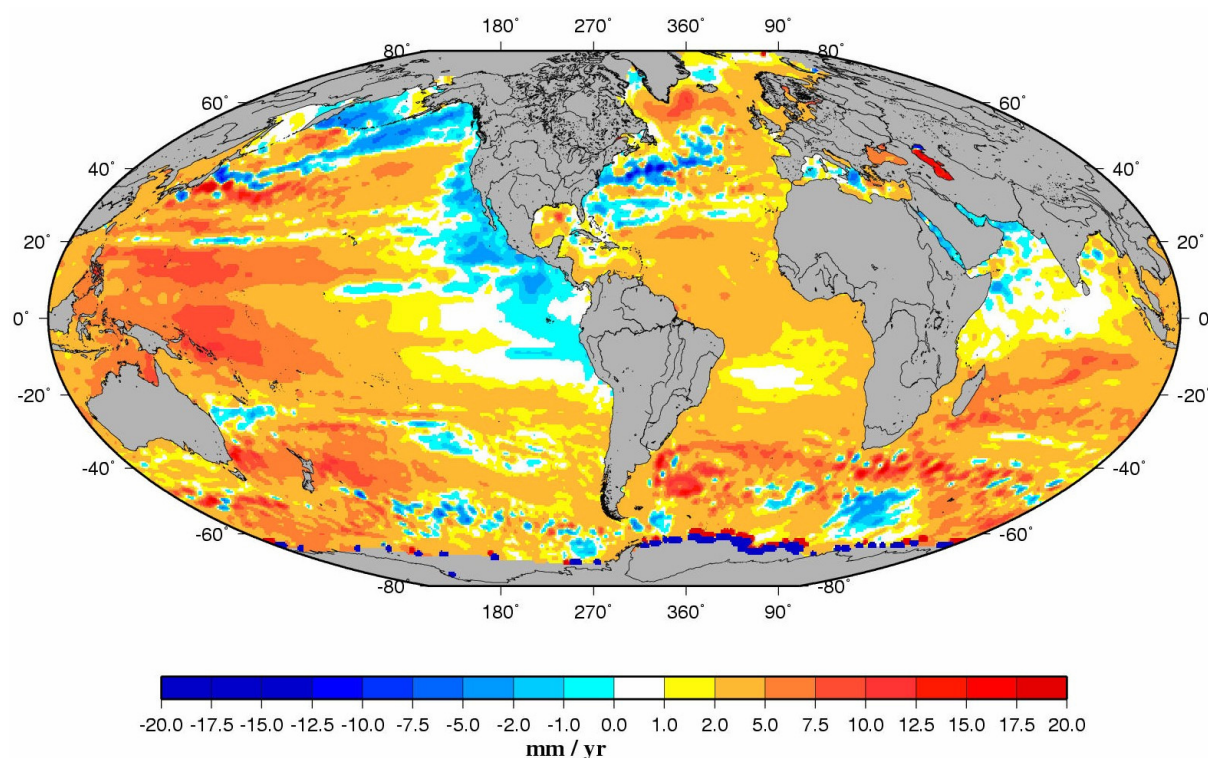
Fig. 8.1 – Carte de la distribution géographique des vitesses de variation du niveau de la mer (1993-2007) d'après Topex/Poseidon et Jason-1. URL : http://www.legos.obs-mip.fr/fr/equipes/gohs/resultats/b1_nivmer1 (consulté le 5 octobre 2008).
