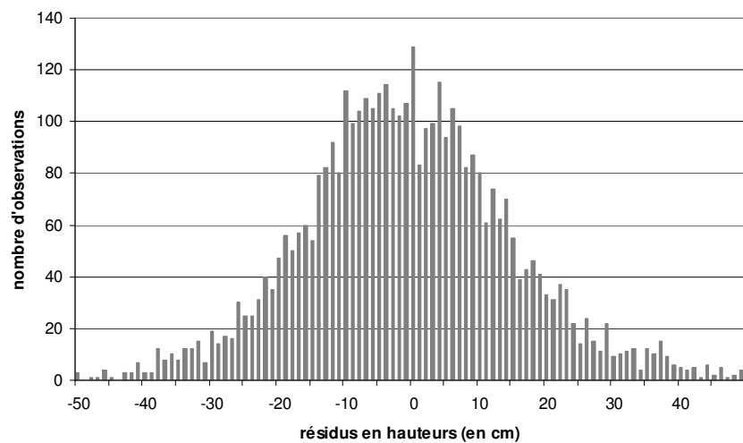
Fig. 7.10.c – Distribution des résidus en hauteurs des PM et BM de 1807 à 1811 (en cm).
