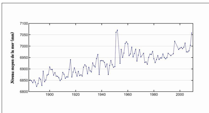
Fig. 2 : série chronologique des moyennes annuelles du totalisateur de Marseille.
