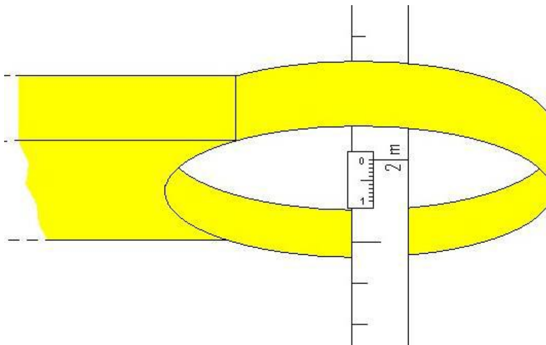
Fig. 20 : lecture sur le ruban porte-sonde par rapport à l'index.
