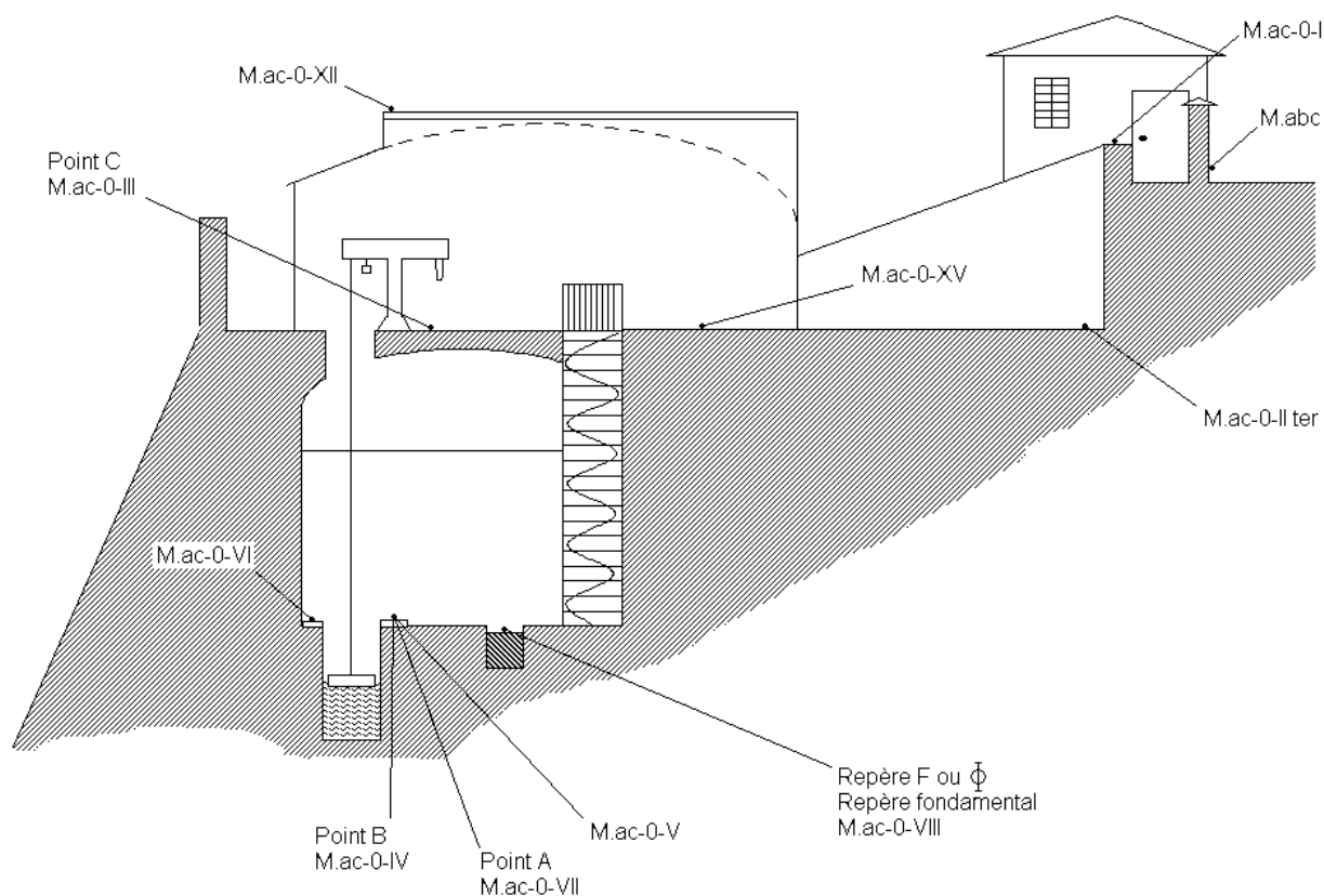
Fig. 26 : repères de nivellement implantés au marégraphe de Marseille.
