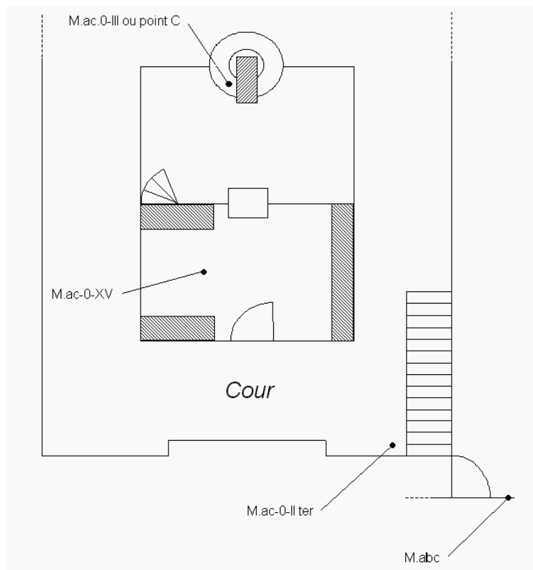
Fig. 25 : rivets de nivellement implantés au rez-de-chaussée.
