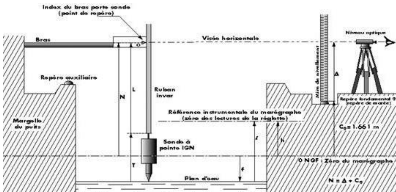
Fig. 27 : description du dispositif de détermination de la hauteur de l'index de lecture de la sonde lumineuse IGN (extrait de Wöppelmann – 1997).
