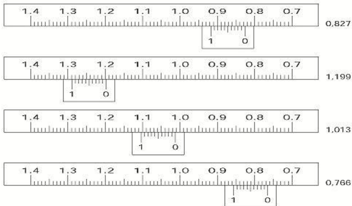
Fig. 18 : exemple de lectures sur la réglette du marégraphe mécanique
